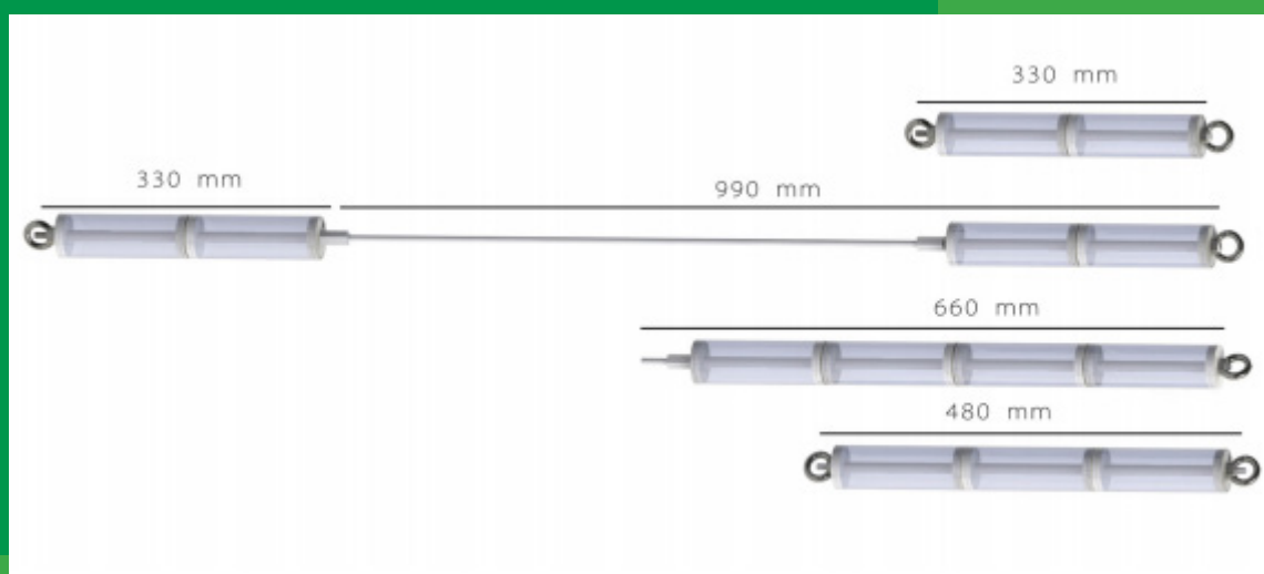
Figure 1 : Matériel nécessaire pour la mise en œuvre des échantillonneurs iFLUX (de gauche à droite : 1 concentration à 1 profondeur ; 1 concentration à 2 profondeurs ; 3 concentrations à 1 profondeur ; 2 concentrations à 1 profondeur)
