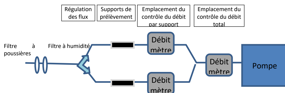
Figure 4 : Schéma de principe d'un prélèvement d'air intérieur et contrôle des débits.
