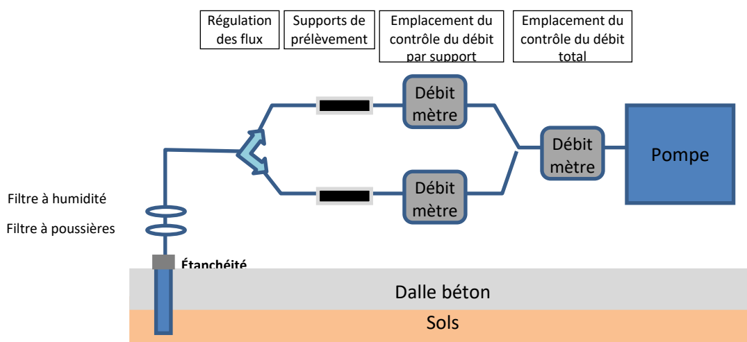
Figure 3 : Schéma de principe d'un prélèvement d'air sous dalle
